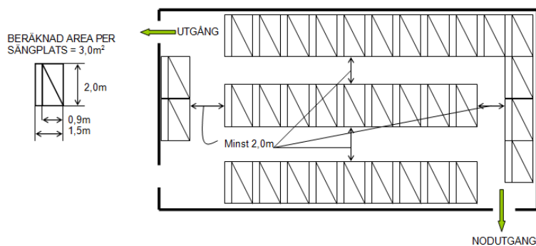
Figur 1 Särskilda utrymningsgångar
